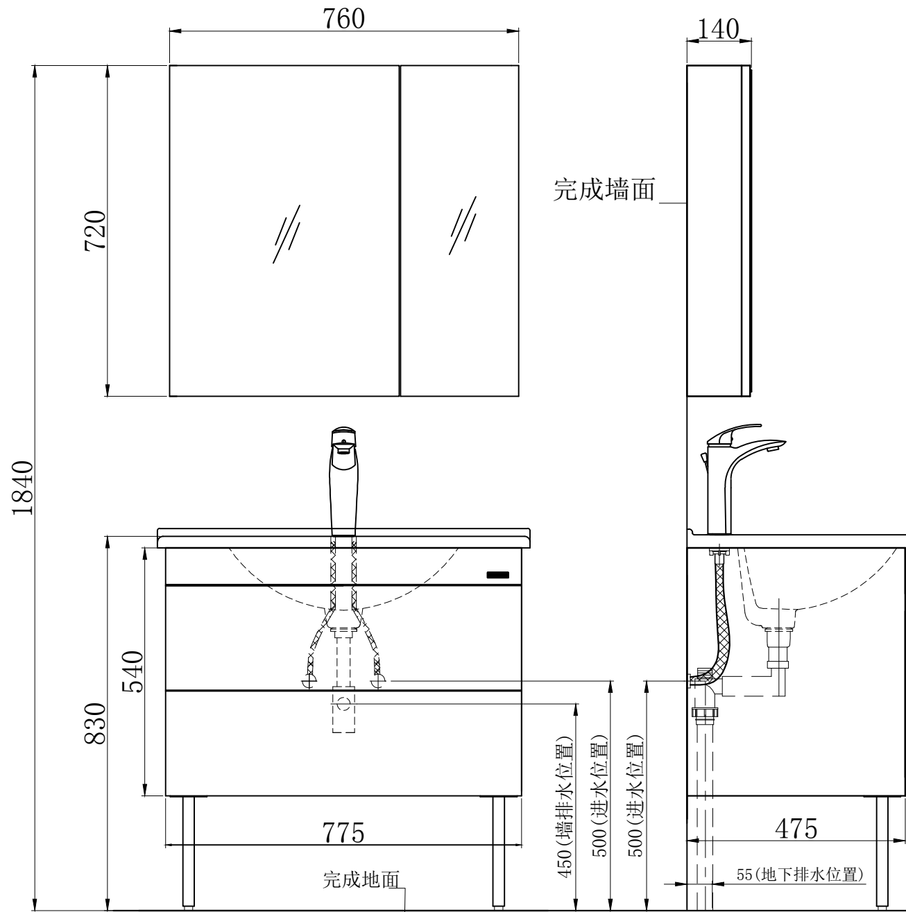
N1D80G10-M 水电安装图 (建议安装尺寸)
