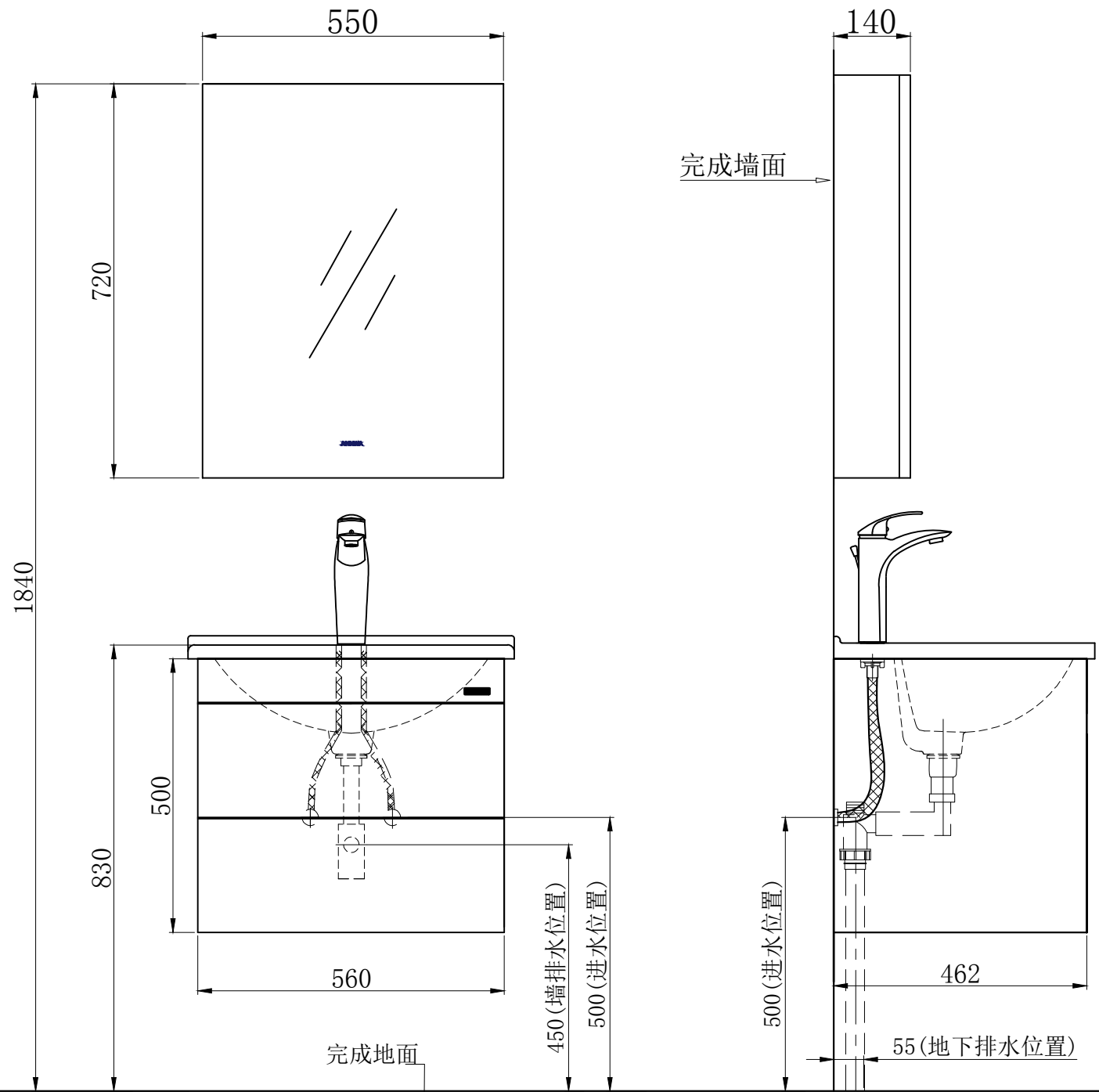
N1D60G10-M 水电安装图 (建议安装尺寸)
