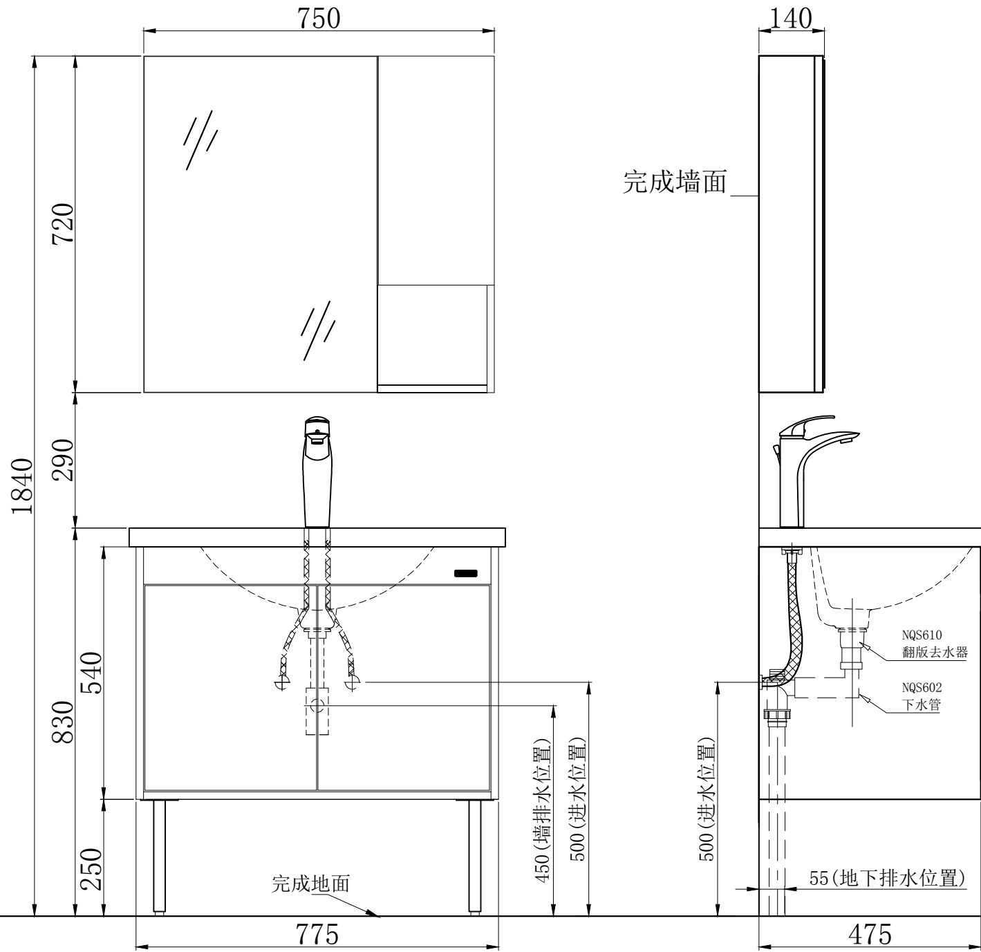
N1D80G10-V 水电安装图 (建议安装尺寸)
