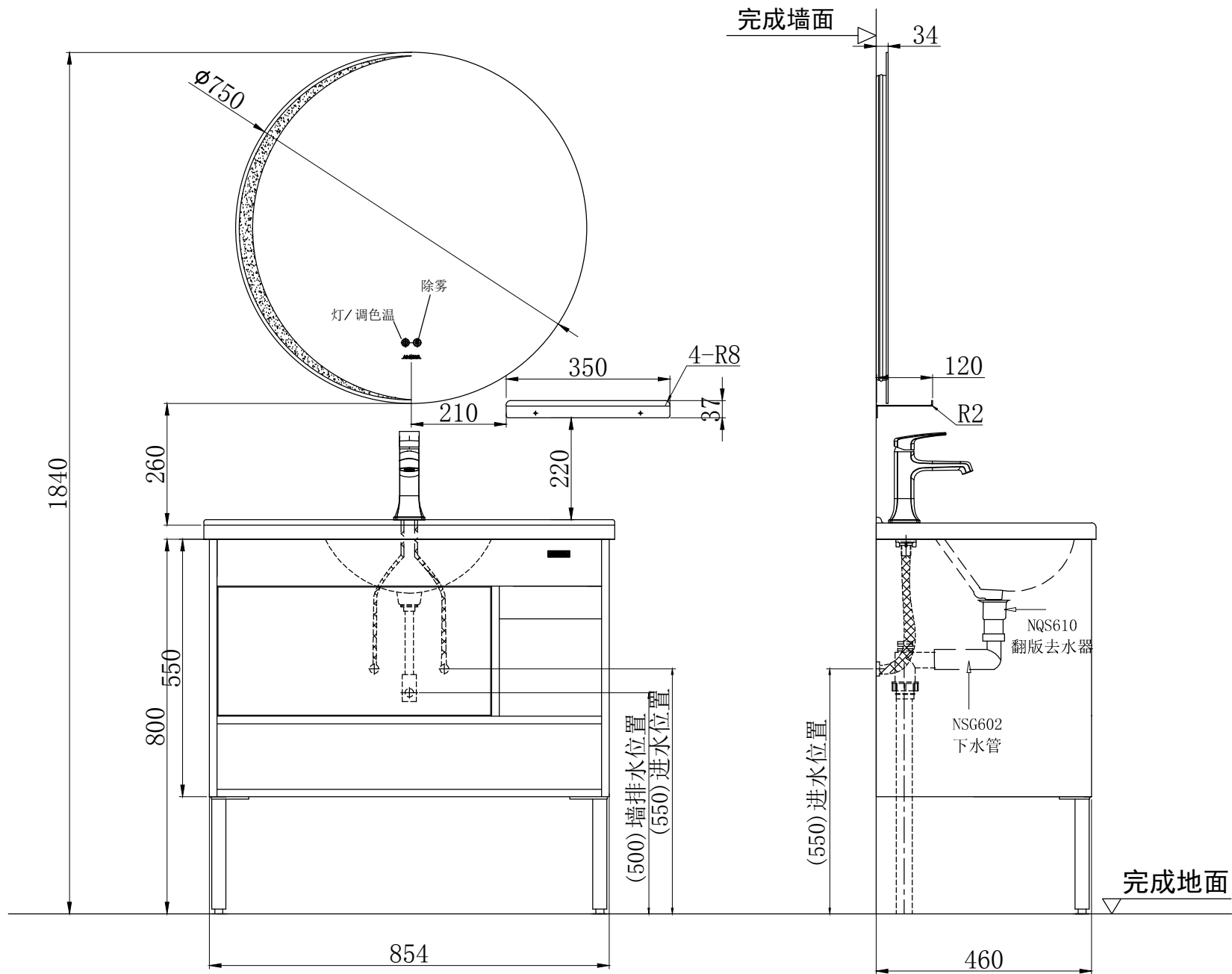
N1D90G10-W 水电安装图 (建议安装尺寸)
