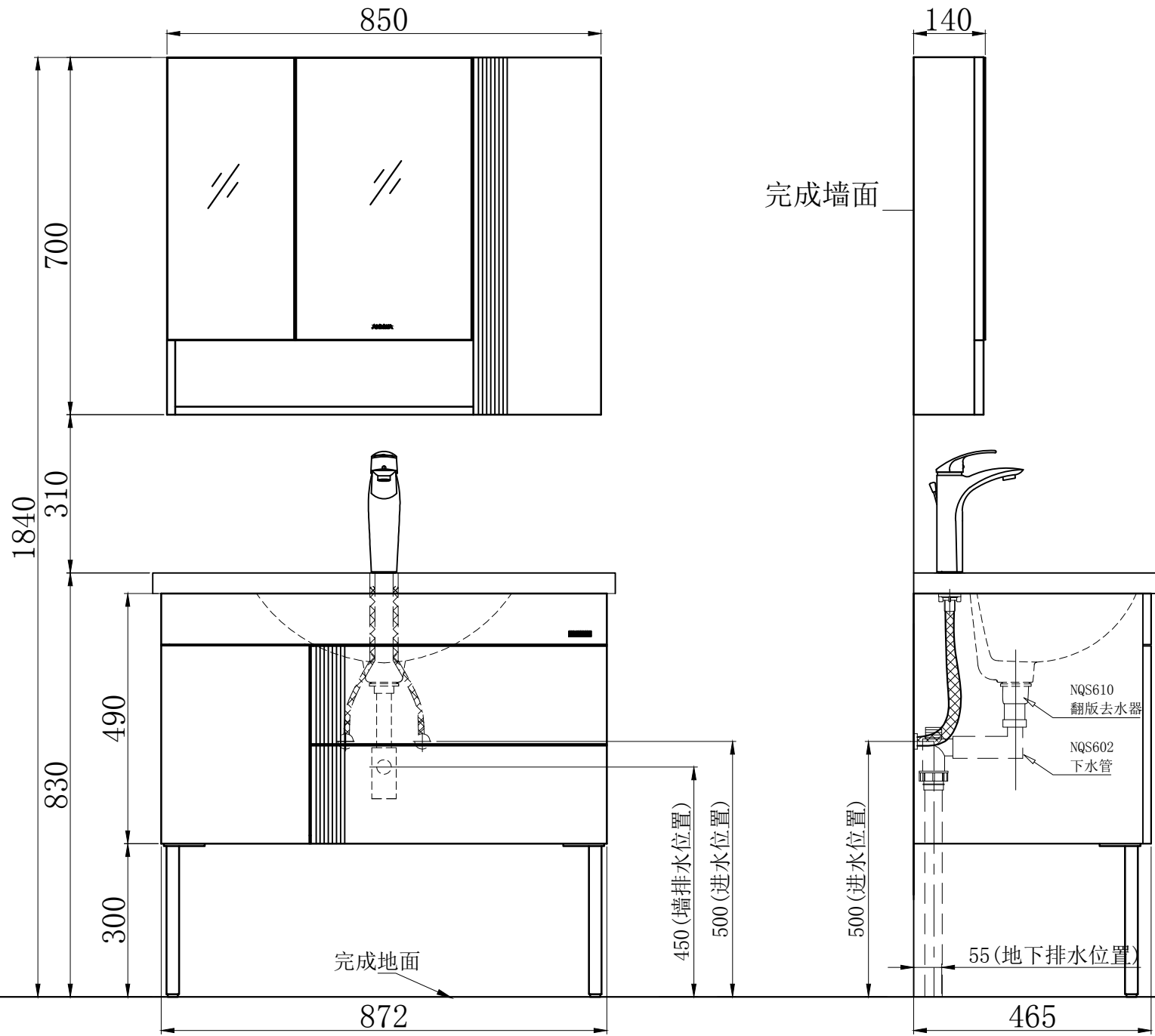
N1H90G03 水电安装图 (建议安装尺寸)
