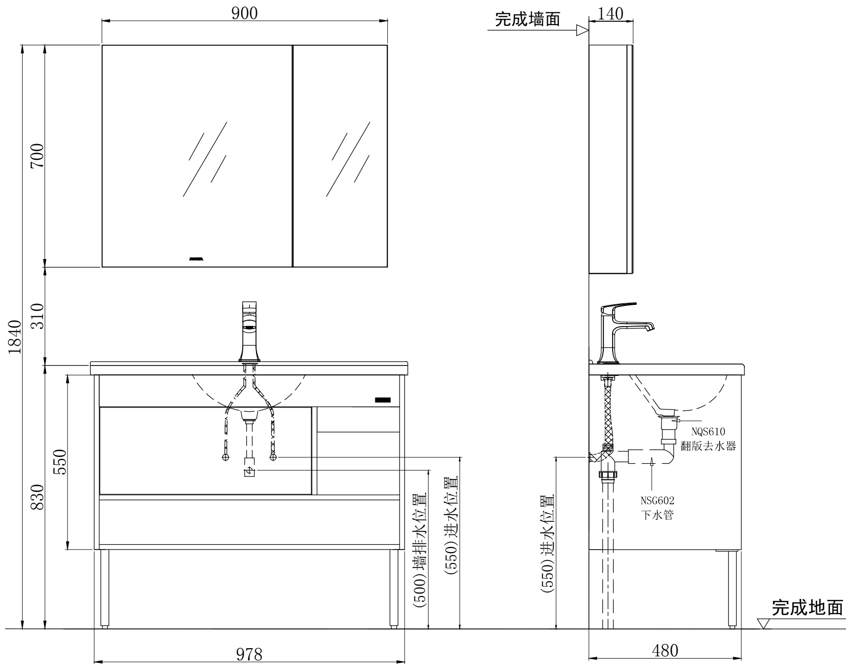
N1D10G10-W 水电安装图 (建议安装尺寸)
