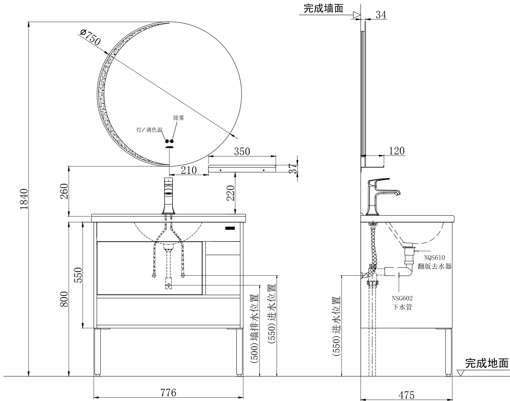
N1D80G10-W 水电安装图 (建议安装尺寸)
