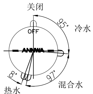
阀芯开启示意图
