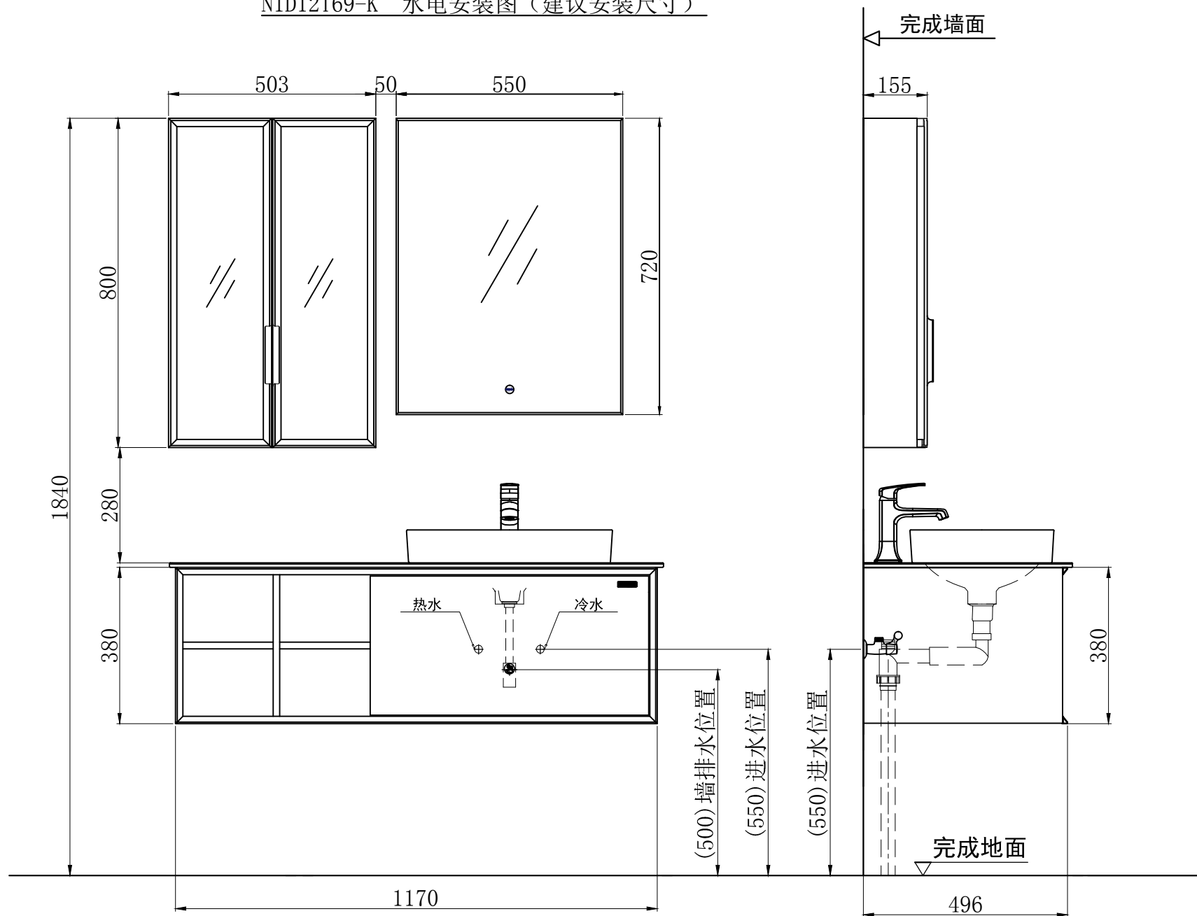
N1D12T69-K 水电安装图 (建议安装尺寸)
