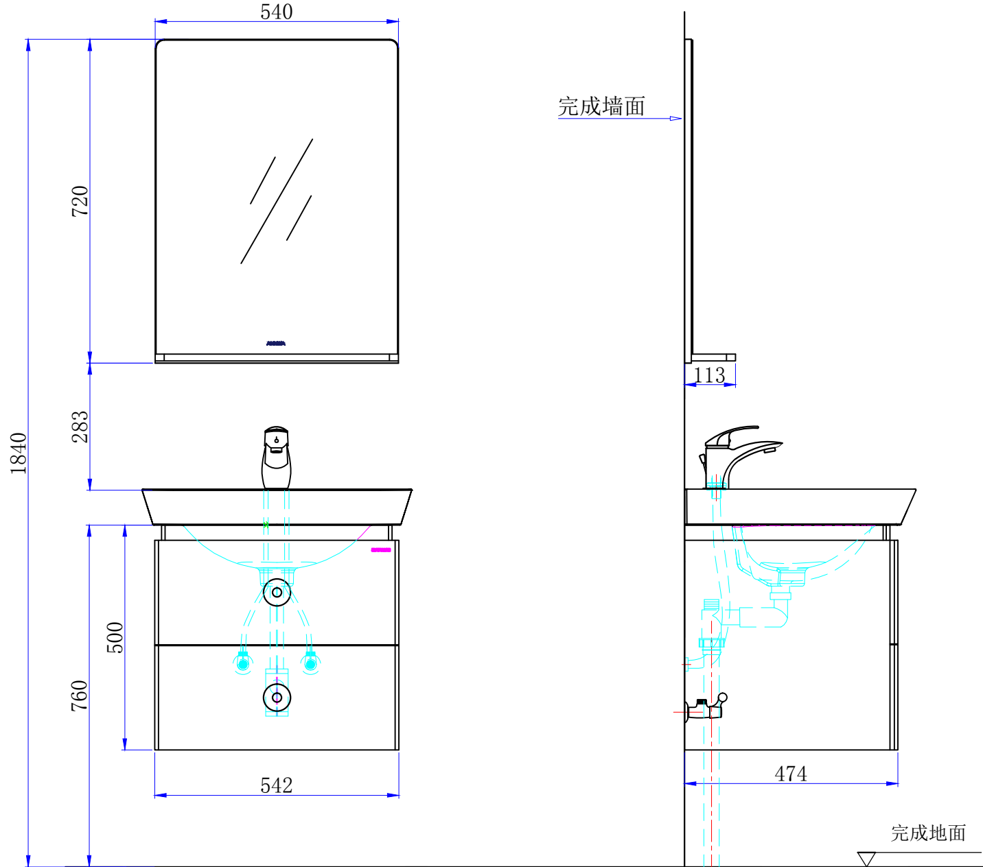
N1P60G07 PVC柜水电安装图（建议安装尺寸）
